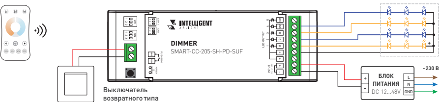
Рис. 4. Схема подключения диммера для управления MIX-нагрузкой
