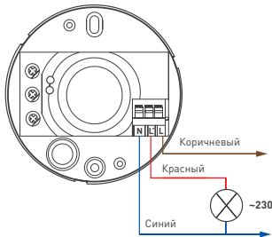
Рисунок 1. Схема подключения датчика движения
