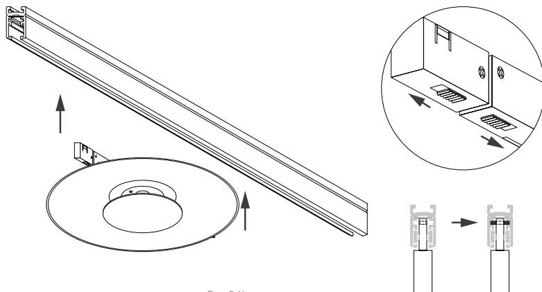
Рис. 2. Установка светильника
