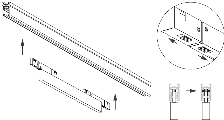
Рис. 2. Установка светильника
