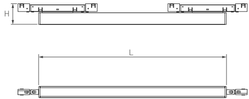
Рис. 1. Чертеж и габаритные размеры
