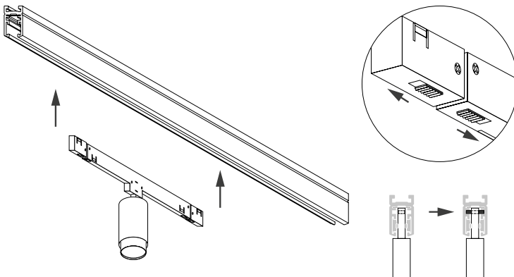
Рис. 2. Установка светильника
