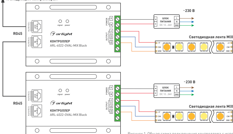
Рисунок 1. Общая схема подключения контроллера с использованием патч-корда для обеспечения синхронной работы контроллеров.
