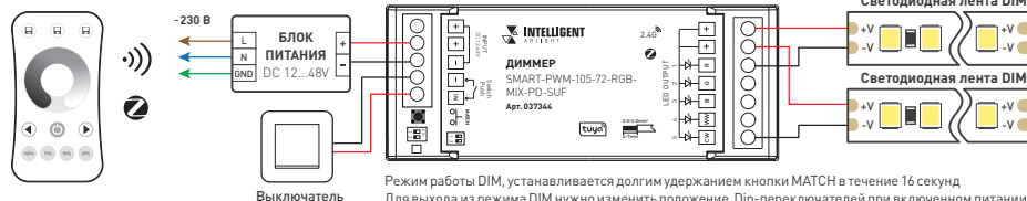
Рис. 1. Схемы подключения диммера SMART-PWM-105-72-RGB-MIX-PD-SUF
